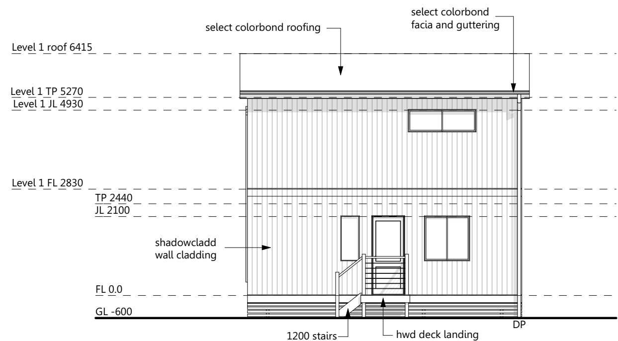
4 Elevation 4 1:100
