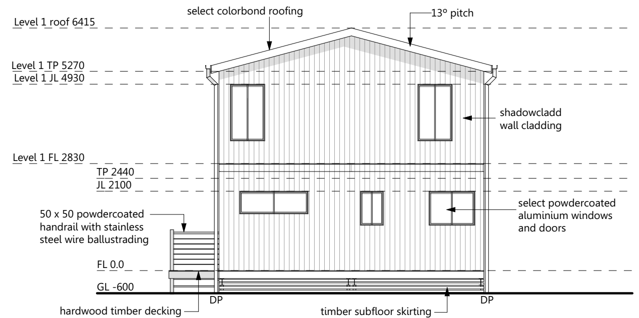
2 Elevation 2 1:100
