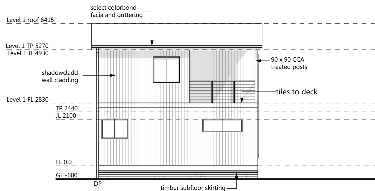
3 Elevation 3 1:100
